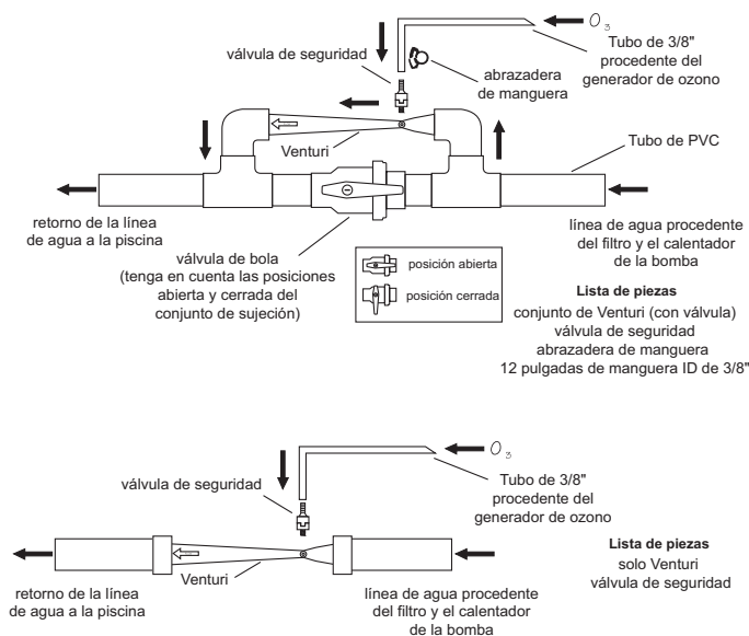
Figura 3 Ejemplos de instalaciones de Venturi
