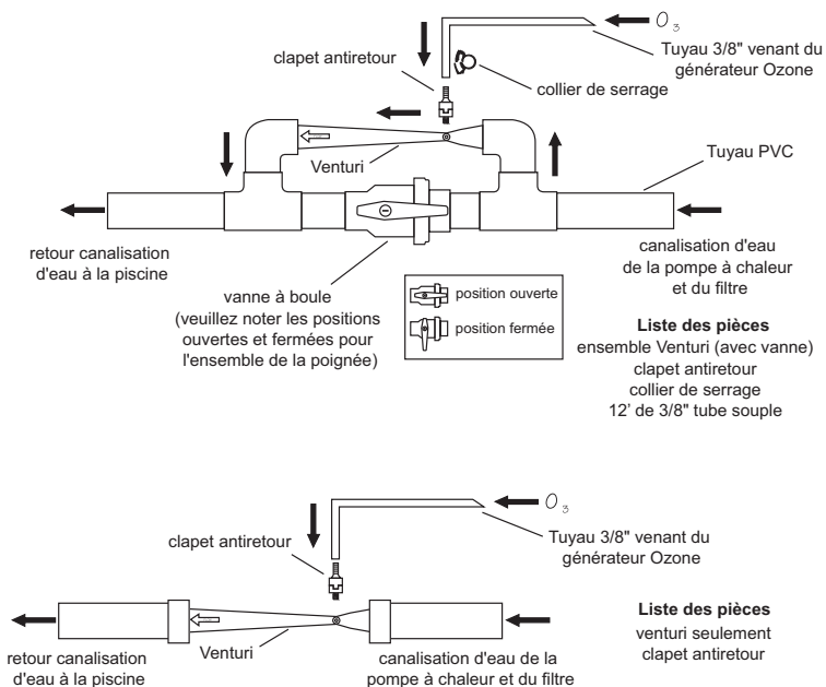
Figure 3 Exemples d'installations Venturi
