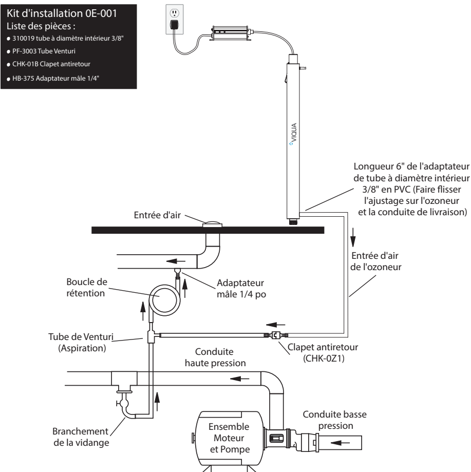
Figure 2 Système à pression différentielle
